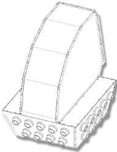
Luftverteilplenum 4-Seiten
